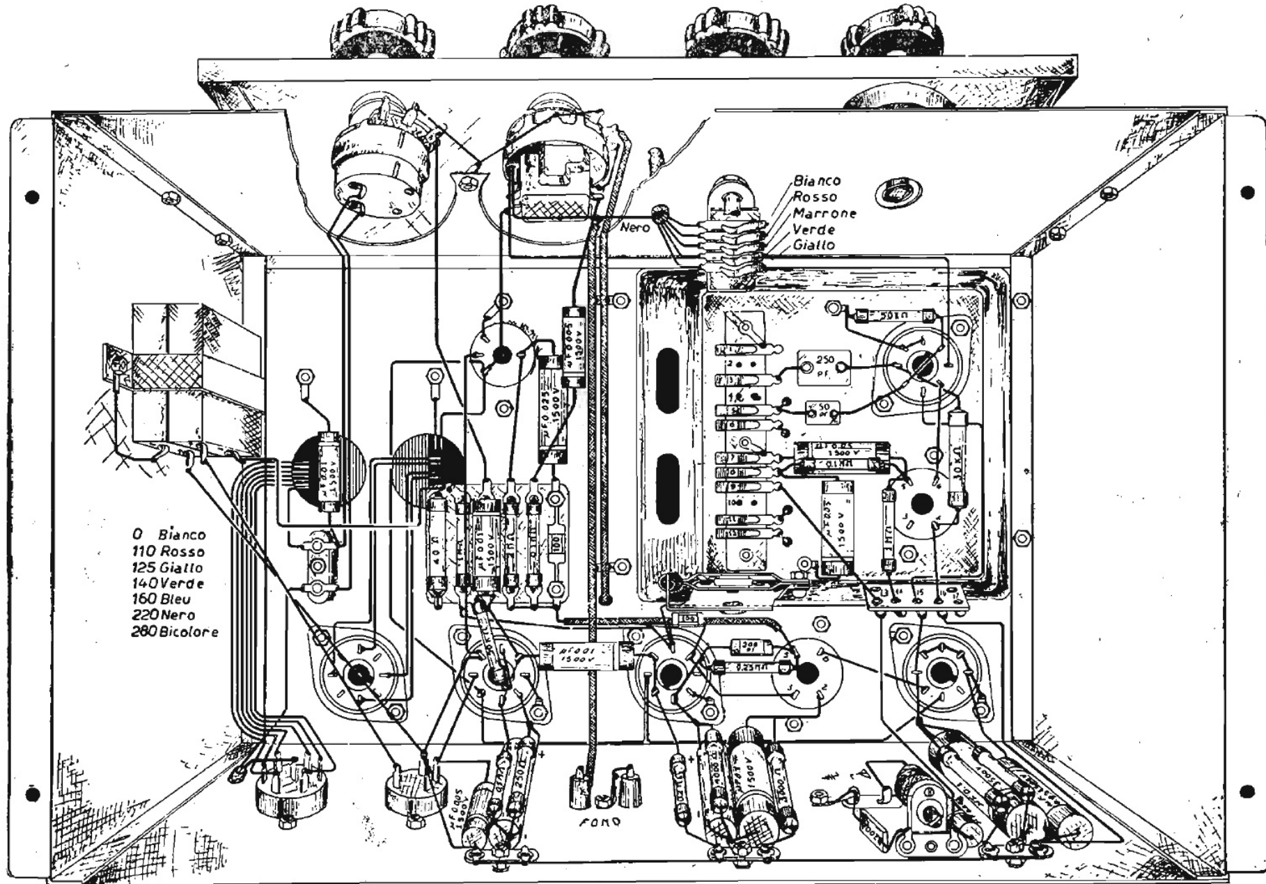
PEBA RADIO . Mod. A/505. Schema di cablaggio.
